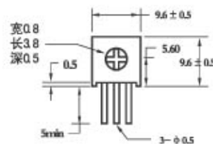
WI112-5(3386C)
