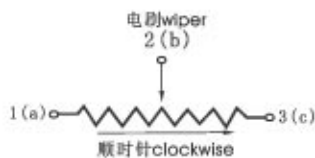
WI112-2(3386F)
